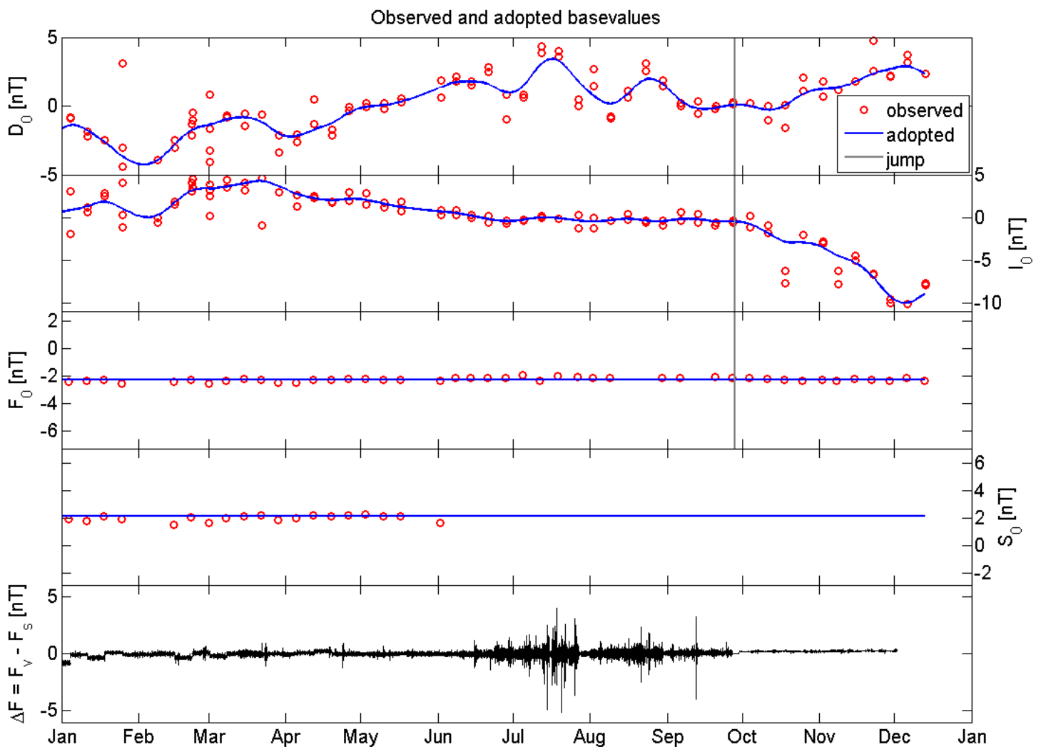
Slika 2.2 – Opažene ( engl. observed ) i prilagođene ( engl. adopted ) kalibracijske vrijednosti za DIDD variometar. Na slici su također prikazani rezultati motrenja s početka prosinca koji su korišteni u izračunu kalibracijskih krivulja za studeni.
