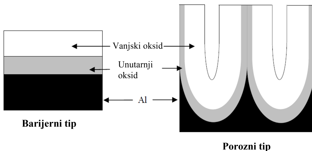
Slika 4.4: Barijerni i porozni tip aluminijskog oksida. Preuzeto i prilagođeno iz [29].
