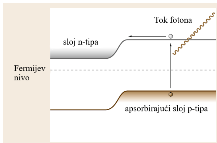
Slika 3.5: Shematski prikaz dijagrama vrpci za p - n spoj fotovoltaika koji prikazuje fotoapsorpciju koja stvara elektron-šupljina par te difuziju elektrona prema spojnici. Preuzeto i prilagođeno iz [14].
