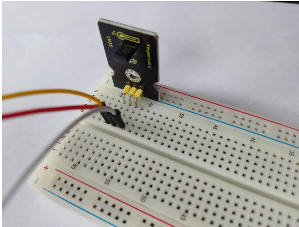
Slika 10 Senzor temperature LM35 spojen na ploču za spajanje komponenti
