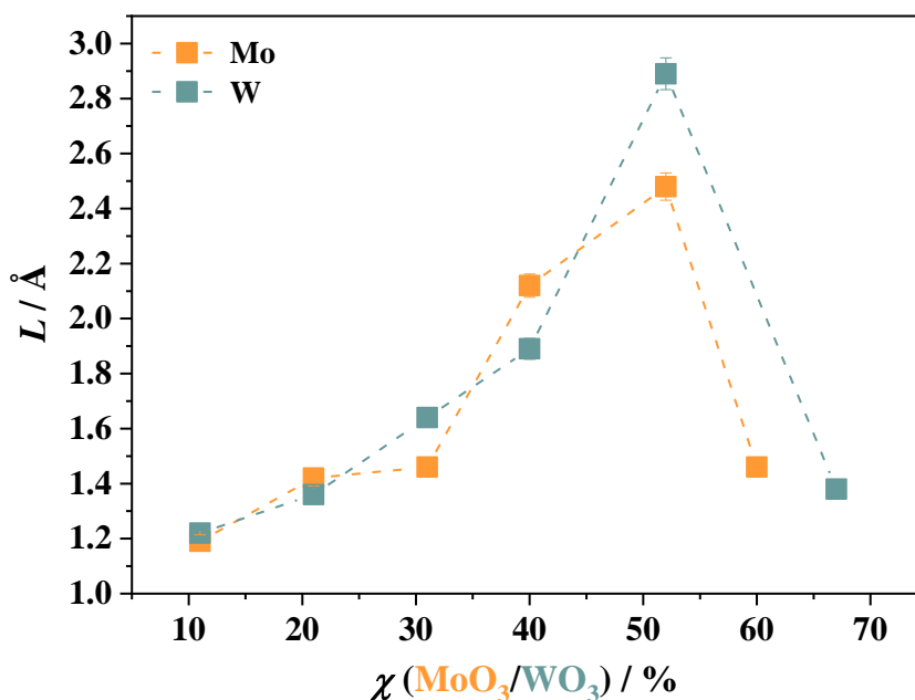
Slika 49. Ovisnost Sidebottomove duljine, L , o udjelu \text{MoO}_3 odnosno \text{WO}_3 za stakla iz serije 2: \chi\text{MoO}_3-(60-\chi)\text{V}_2\text{O}_5-40\text{P}_2\text{O}_5 , \chi = 11 - 60 \% i serije 3: \chi\text{WO}_3-(60-\chi)\text{V}_2\text{O}_5-40\text{P}_2\text{O}_5 , \chi = 11 - 67 \% .
