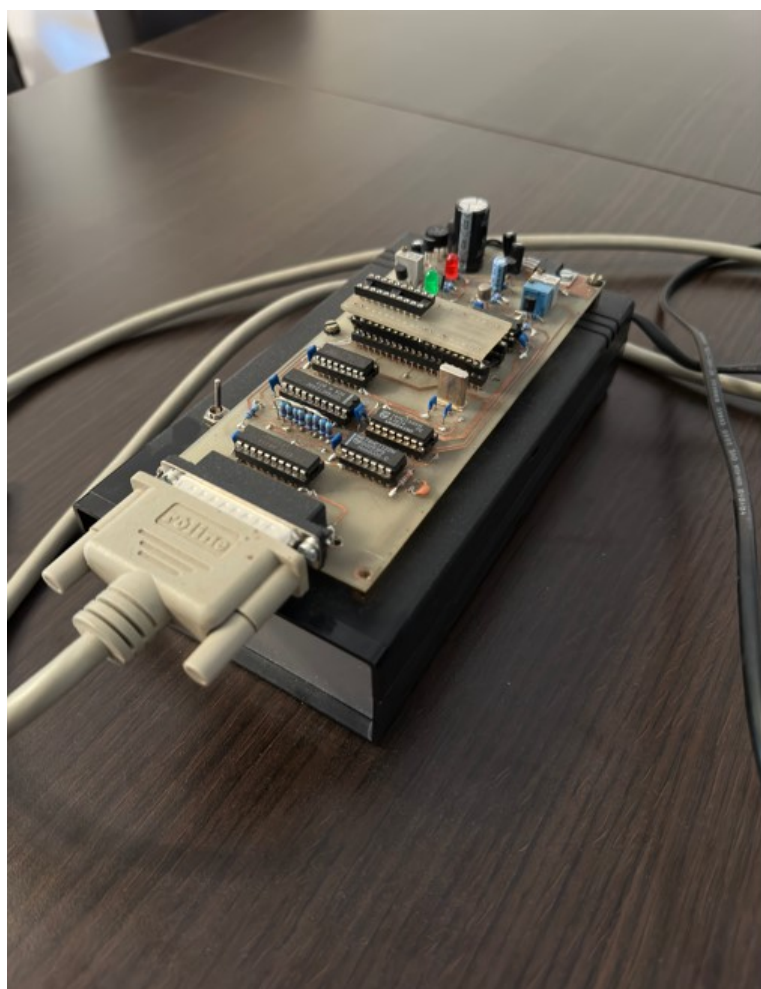
Slika 2.7: Programator PG302
