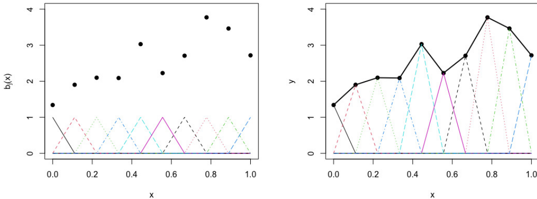
Slika 2.2: Lijevi graf prikazuje primjer baze šatorskih funkcija za interpolaciju podataka prikazanih crnim točkama. Svaka od obojenih linija predstavlja pojedina šatorsku funkciju koja doseže svoj maksimum od 1 na x -osi kod jedne od točaka. Desni graf ilustrira postupak u kojem se svaka bazna funkcija množi odgovarajućim koeficijentom, a zatim se rezultati zbrajaju kako bi se formirala konačna interpolacija, prikazana debljom crnom linijom.
