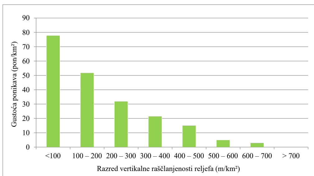
Slika 20. Gustoća ponikava po razredima vertikalne raščlanjenosti reljefa
