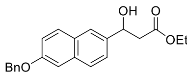
rac-3
