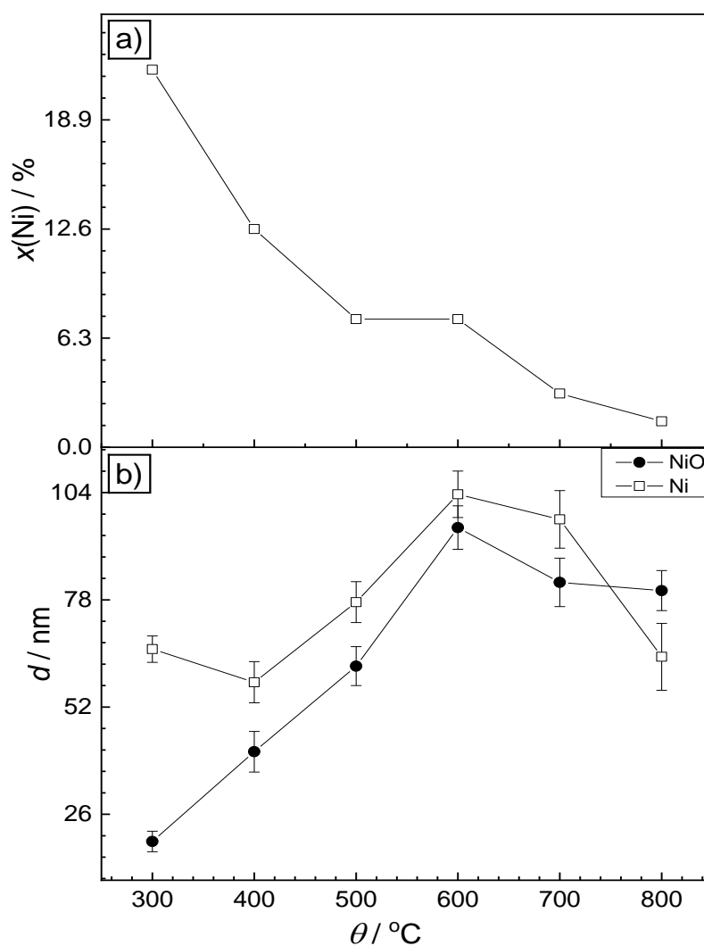
Slika 5.46. a) Množinski udio nastale Ni faze u procesu termičkog raspada niklovog(II) acetata tetrahidrata u ovisnosti o temperaturi, b) veličine kristalita korespondentnih Ni i NiO faza na temelju XRD mjerenja.
