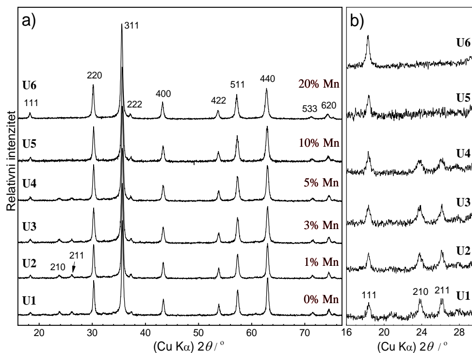
Slika 5.33. Rendgenski difraktogrami pripremljenih uzoraka U1 – U6 termičkim raspadom smjese \text{Fe}(\text{acac})_3 i \text{Mn}(\text{acac})_2 uz naznačeni množinski udio mangana u odnosu na željezo x(\text{Mn}/\text{Fe}) .
