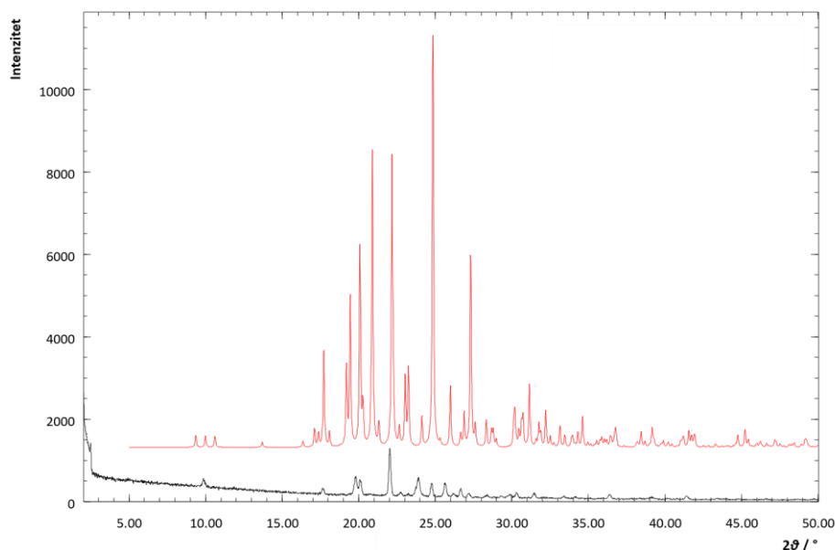
Slika D21. Difraktogram sintetiziranog praškastog uzorka soli (HNZ)ClO 4 (crno) te generiranog pomoću programa Mercury (crveno).
