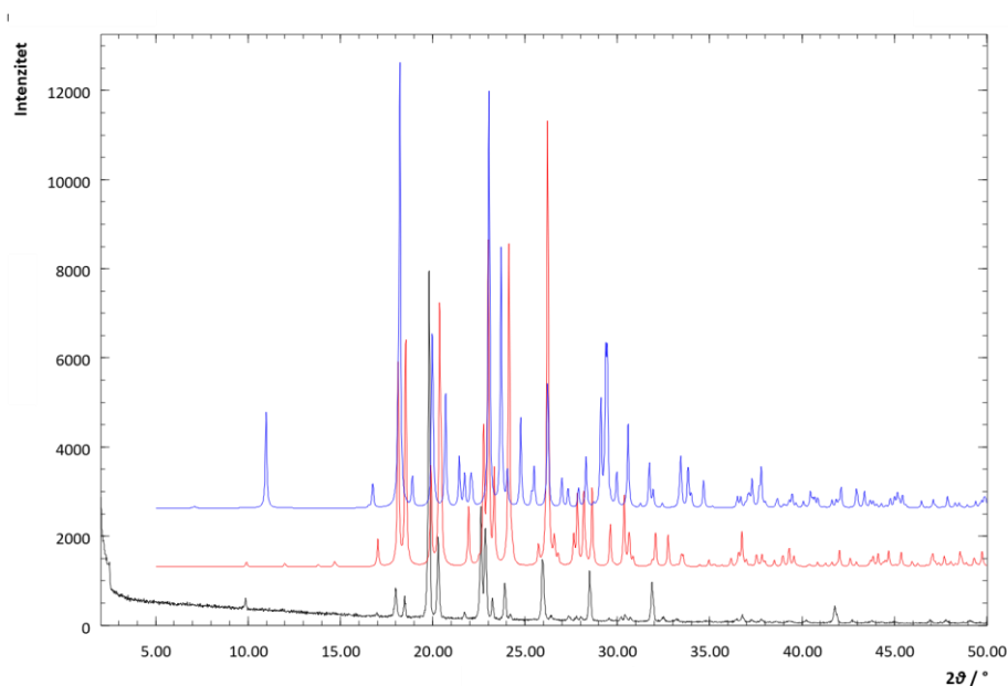
Slika D20. Difraktogram sintetiziranog praškastog uzorka soli (HINZ)ClO 4 (crno), uzorka priređenog monokristala (crveno) te monohidratne perkloratne soli INZ 57 (plavo) generiranog pomoću programa Mercury. Razlike u položajima i intenzitetima difrakcijskih maksimuma mogu se pripisati različitim temperaturama snimanja difraktograma praha i jediničnog kristala.
