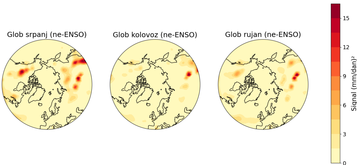
Slika 3.14 Polja signala oborine [\text{mm/dan}]^2 dobivena eksperimentom Glob u ne-ENSO godinama.
