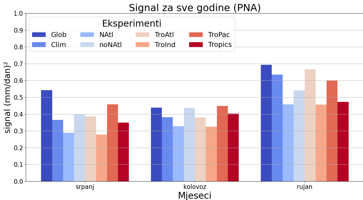
Slika 3.37 Signal oborine [mm/dan] 2 u ljetnim mjesecima usrednjen preko područja PNA za sve godine.
