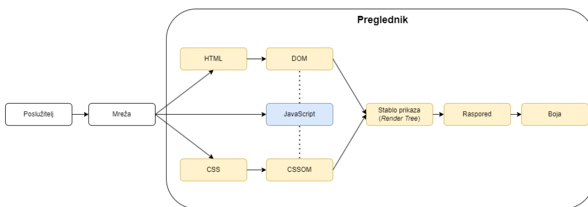
Slika 1.2: Rad preglednika
