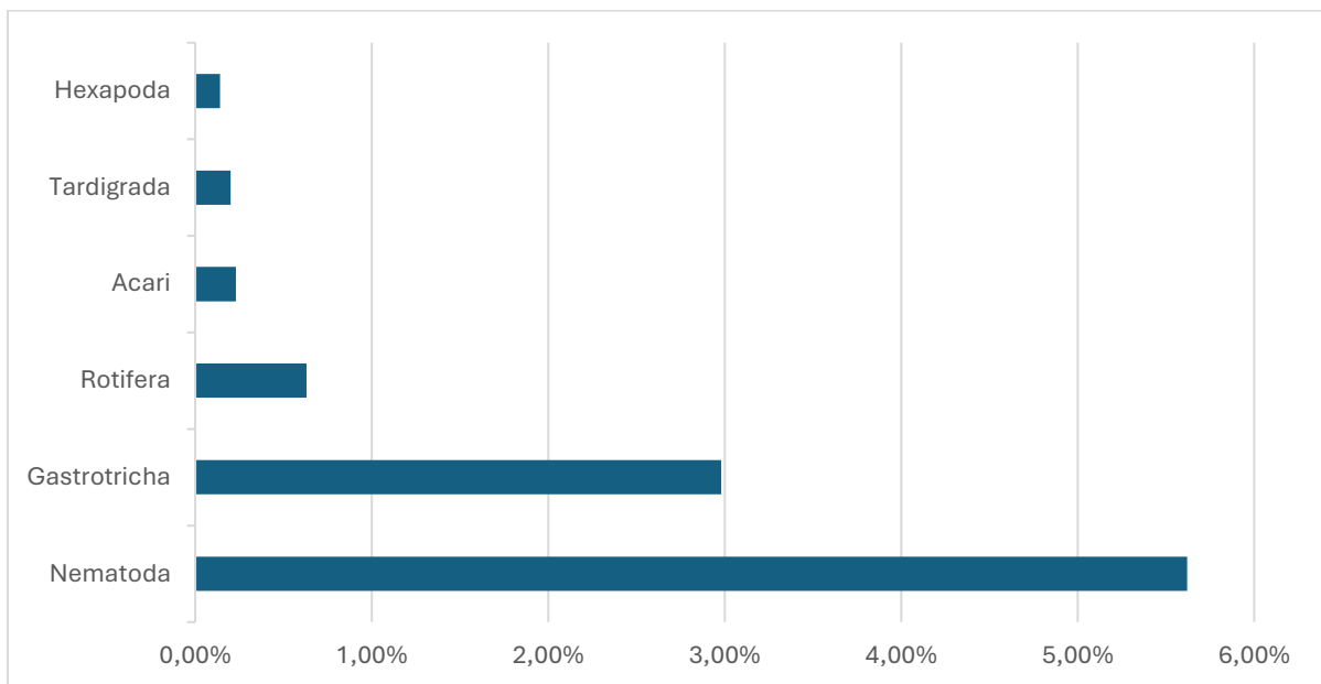
Slika 15. Srednje vrijednosti udjela brojnosti skupina mikro-beskraljješnjaka u analiziranim uzorcima tla.
