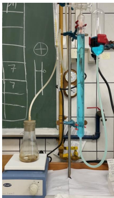
Slika 6: Scheiblerova aparatura za kalcimetriju.
