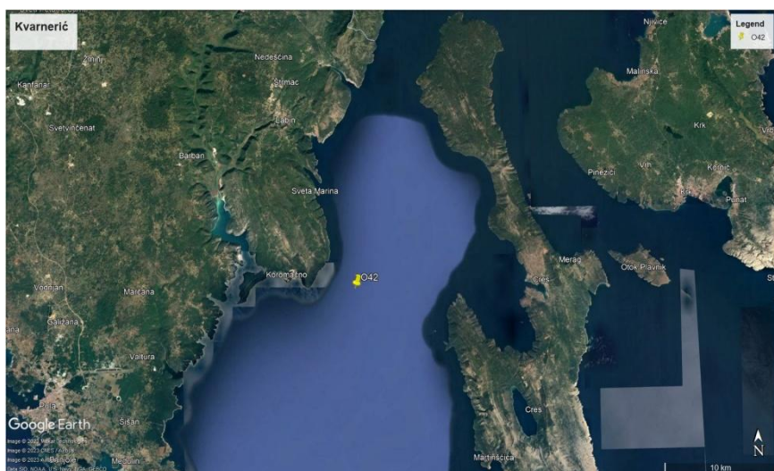
Slika 1: Satelitska snimka područja uzorkovanja uzorka 042 (Izvor: Google Earth).
