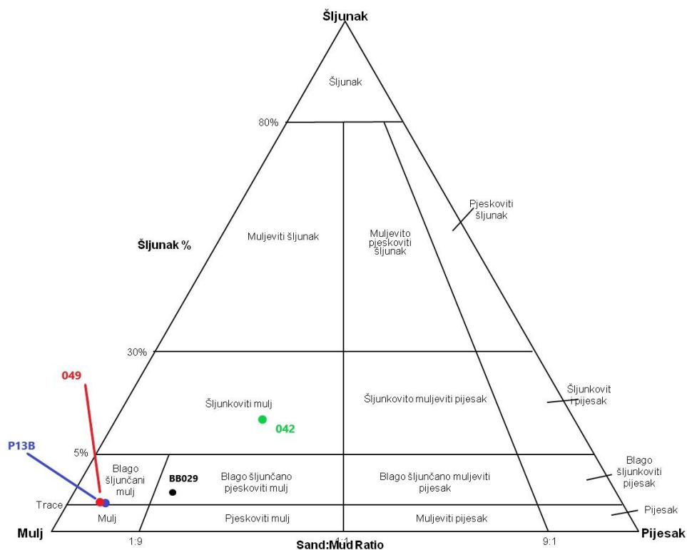
Slika 7: Tipovi sedimenta za uzorke BB029, P13B, 049 i 042.
