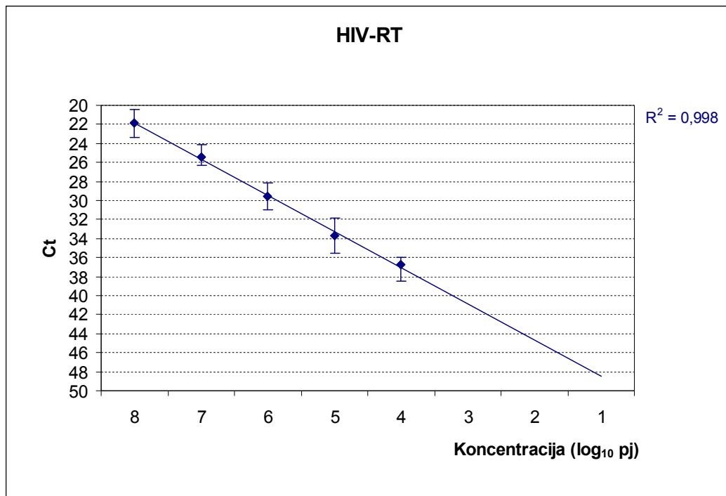
Slika 18. Srednja vrijednost Ct za HIV-RT u tri PERT-testa ( \bar{X}_{n_r} , Tablica 9.). Stupci pogreške predstavljaju raspon Ct iz svih testiranja pojedine koncentracije RT. Povučeni je regresijski pravac i određen koeficijent determinacije.
