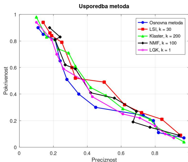
Slika 3.1: Usporedba metoda
