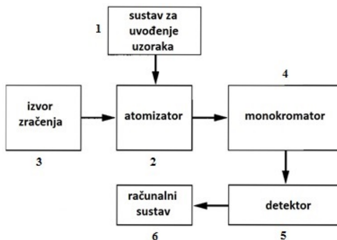
Slika 8. Shematski prikaz atomskog apsorpcijskog spektrometra
