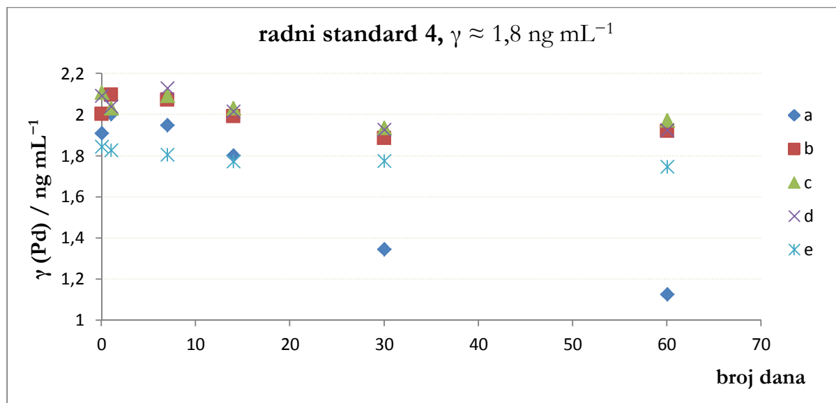
Slika 14. Stabilnost radnih standarda paladija, a) 5 % HNO 3 (v/v), b) 5 % HNO 3 / 1 % HCl (v/v), c) 5 % HNO 3 / 2 % HCl (v/v), d) 5 % HNO 3 / 5 % HCl (v/v) i e) 1 % HCl (v/v)
