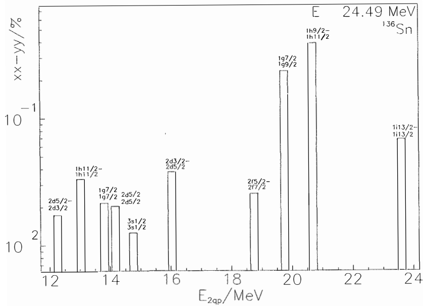
Slika 12: Struktura rezonantnog GT vrha na E = 24.49 MeV , za 136 Sn.
