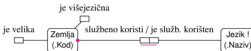
Slika 3.3: Object Role Modeling dijagram
