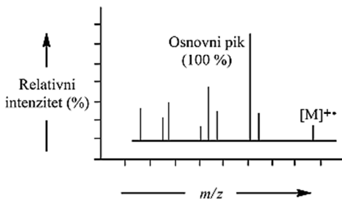
Slika 2.39. Maseni spektar
