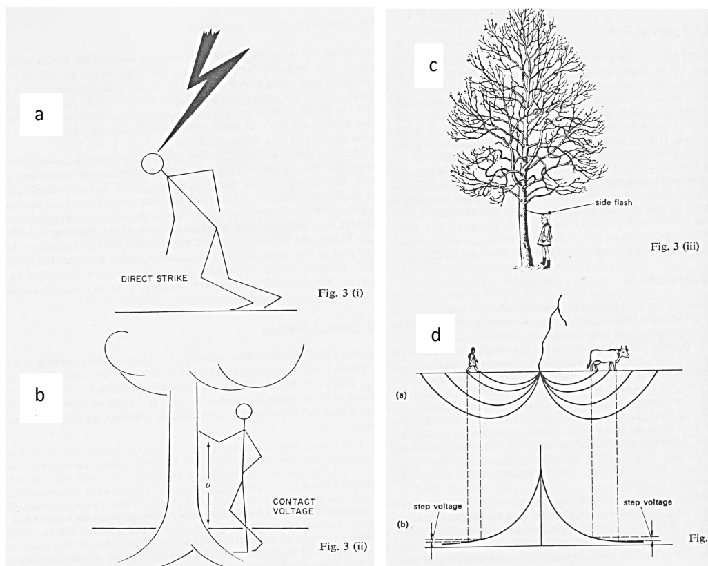
Slika 56:a) direktni udar; b) kontakti napon; c) postrani udarac; d) step-napon d_{(a)} distribucija struje, d_{(b)} pad napona duž površine zemlje [29.]
