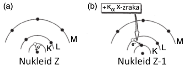
Slika 2.3: (a) Elektronski uhvat iz K ljuske. (b) Pomak elektrona iz L u K ljusku rezultirajući emisijom X zraka [7]
