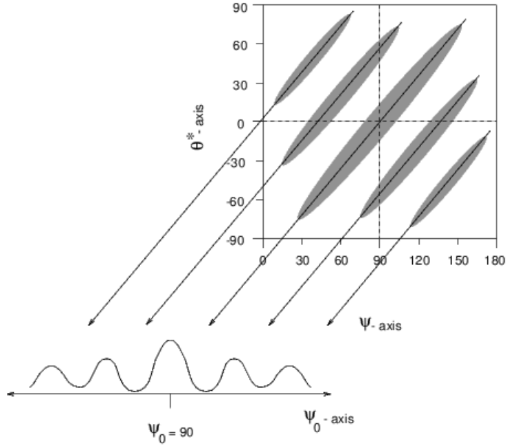
Slika 2.27: Skica pruga u \theta^* - \psi kutnom korelacijskom spektru te projekcija podataka na os \psi pod kutem paralelnim tim prugama, za \theta^* = 0^\circ opisanih Legendrovim polinomom. Spin prikazan na ovoj skici je paran jer se maksimum polinoma pojavljuje na \psi = 90^\circ , dok bi spin bio neparan kad bi polinom imao minimum [82].
