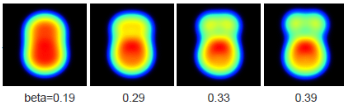
Slika 1.5: Intrinzične distribucije gustoće AMD računa za jezgru ^{24}\text{Mg} [45].
