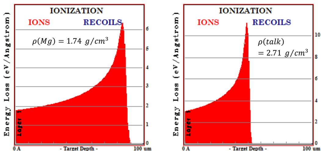
Slika 2.3. Raspodjela elektronskog kočenja (ionizacije) protona energije 2.41 MeV-a u magneziju (lijevo) i mineralu talku ( Mg_3Si_4O_{10}(OH)_2 ) (desno) u ovisnosti o dubini simulirane pomoću SRIM programa [Zie08]. Vidi se da je zaustavna moć veća u materijalu veće gustoće, tj. u talku.
