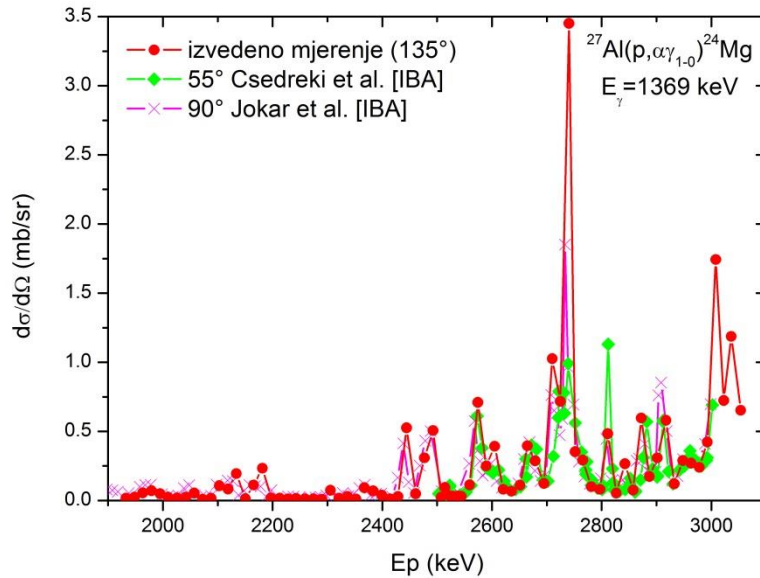
Slika 3.35. Usporedba izmjenjenog diferencijalnog udarnog presjeka za produkciju gama-zračenja na 1369 keV-a iz ^{27}\text{Al}(p, \alpha\gamma)^{24}\text{Mg} reakcije s podacima od Csedreki et al. i Jokar et al. koji su naknadno dostupni u bazi podataka [IBA].
