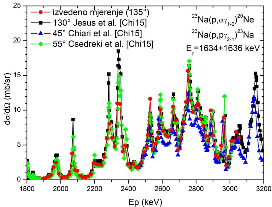
Slika 3.23. Usporedba izmjenog diferencijalnog udarnog presjeka za produkciju gama-zračenja na 1634+1636 keV-a iz reakcija ^{23}\text{Na}(p,\alpha\gamma)^{20}\text{Ne} i ^{23}\text{Na}(p,p'\gamma)^{23}\text{Na} s podacima naknadno dostupnim u bazi podataka [IBA] i uključenih u zajedničku publikaciju [Chi15] mjerenih na sličanom kutu.
