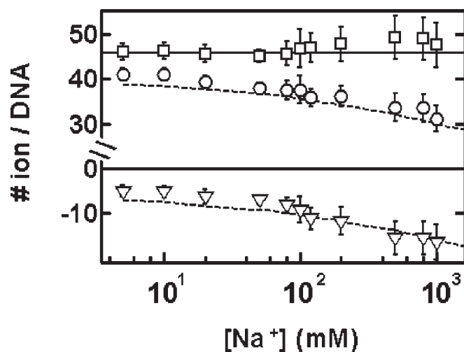
Slika 1.29: Neutralizacija 24bp DNA (-46 naboja) asocijacijom \text{Na}^+ ( \circ ) i osiromašenjem aniona ( \nabla ). Asociirani natrijevi ioni uvećani za istisnute anione daju ukupni naboj ionske atmosfere ( \square , puna linija +46). Rezultati su uspoređeni s predviđanjem PB teorije za jednovalentne ione (isprekidane crte). Preuzeto iz [50].
