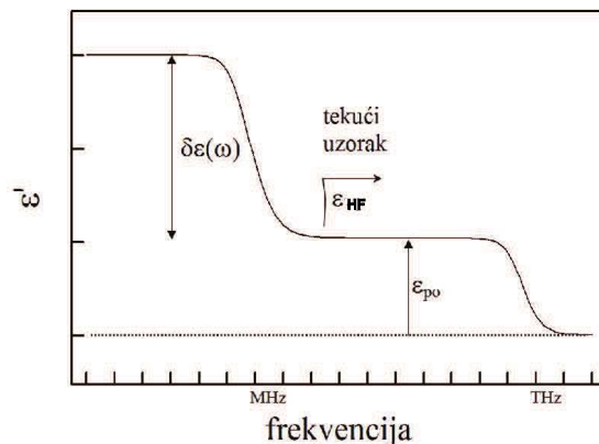
Slika 2.5: Puna crta prikazuje vrijednost realnog dijela dielektrične funkcije uzorka \epsilon_{exp} . Točkasta crta prikazuje vrijednost dielektrične konstante vakuuma, tj. vrijednost 1. Vrijednost dielektrične funkcije istraživanog uzorka \delta\epsilon(\omega) i vrijednost dielektrične funkcije za frekvencije veće od eksperimentalno uočljivih \epsilon_{HF} su obilježene na slici.
