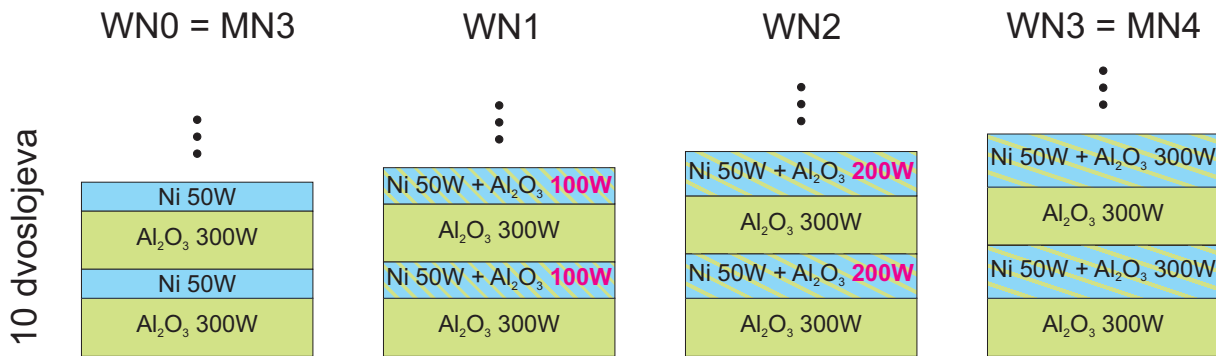
Slika 4.20: Shematski prikaz deponiranja serije uzoraka s različitim udjelom matrice Al 2 O 3 u miješanom sloju.
