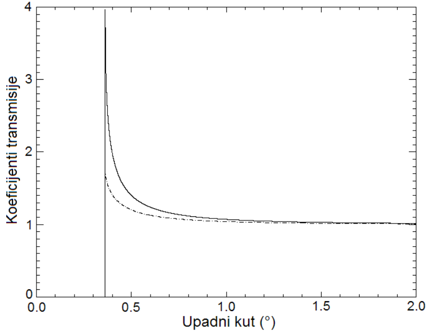
Slika 3.8: Kočificijenti transmisije za idealnu (puna linija) i realnu (isprekidana linija) površinu ( \zeta = 5 nm). Iz [73].
