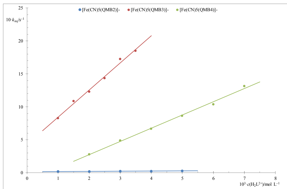
Slika 28. Ovisnost k_{mj} o koncentraciji N,N' -supstituiranog bis(piridinijski-aldoksim) liganda za reakciju nastajanja pentacijano(bis(piridinijski-aldoksim))ferat(II)-kompleksa.
