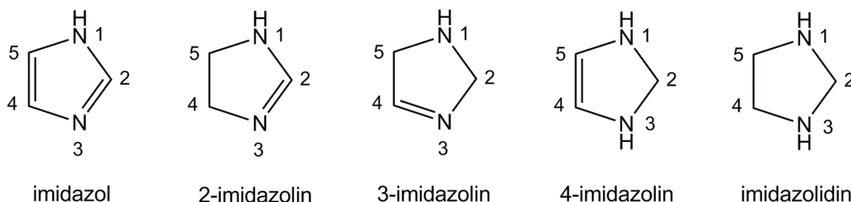
Slika 3. Strukturne formule imidazola i produkata njegove redukcije.
