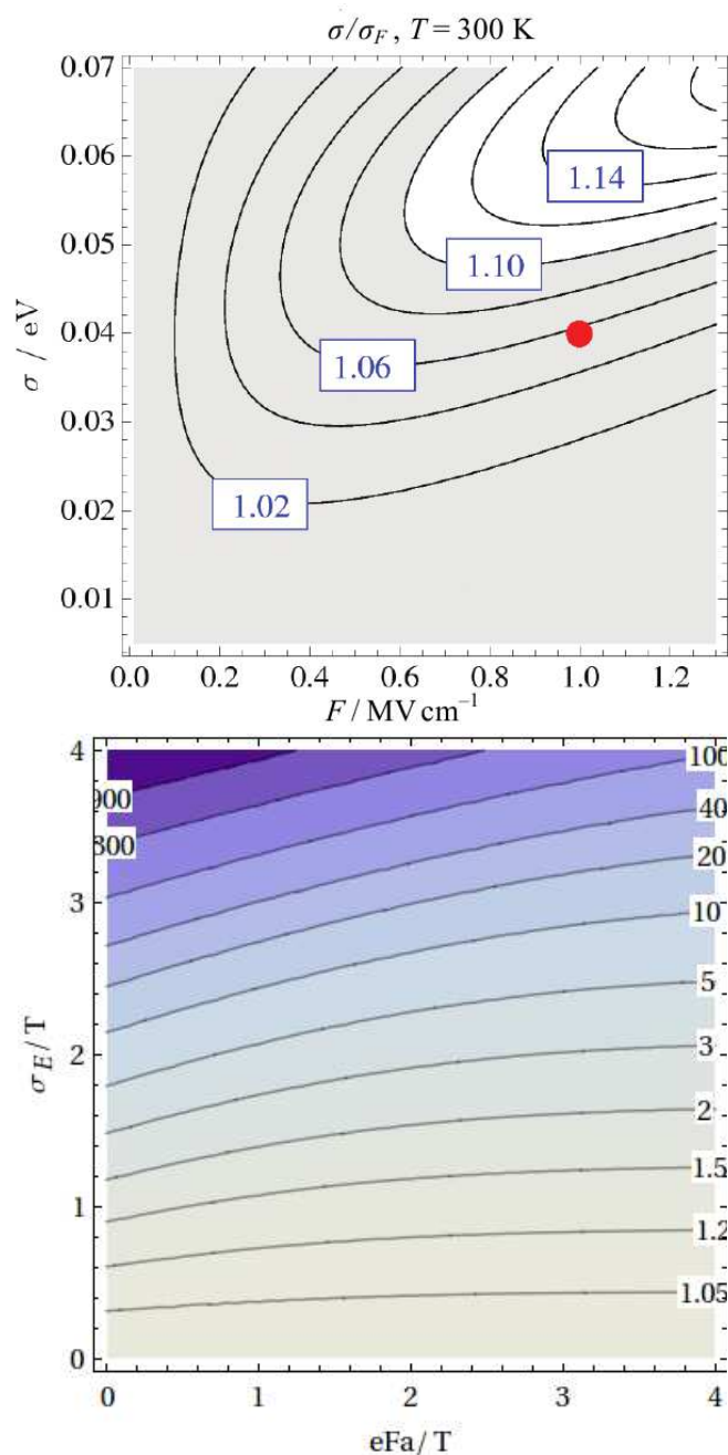
Slika 4.25: Gore: Omjer širine raspodjele O(E) pri stacionarnom toku, i širine raspodjele g(E) , \sigma_F / \sigma_E , u ovisnosti o jačini nereda i jačini polja. Crvena točka odgovara parametrima raspodjele O(E) prikazane na slici 4.23 (b). Dolje: Omjer mobilnosti dobivene supstitucijom stacionarnih koncentracija, n_i , srednjom raspodjelom, n(E) , jed. (4.37), i mobilnosti dobivene rješavanjem glavne jednadžbe.
