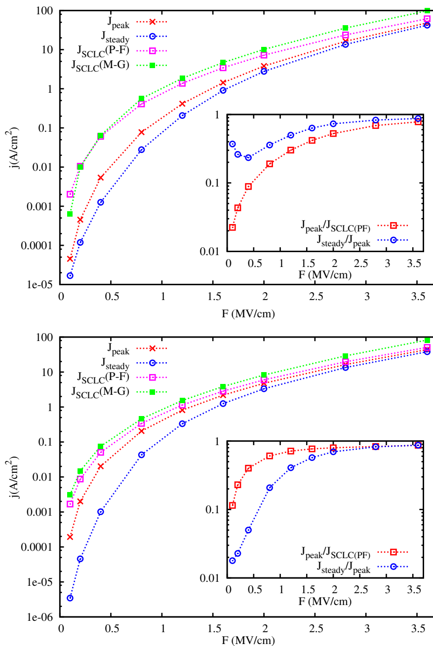
Slika 5.20: Maksimumi tranzijentne struje, J_{\text{peak}} , i konačni iznosi struje, J_{\text{steady}} , s tranzijenata na slici 5.14. Gore je predstavljen slučaj \sigma_E = E_T = 2T i E_c = -2\sigma_E , a dolje slučaj \sigma_E = E_T = 3T i E_c = -3.5\sigma_E . ‘ J_{\text{SCLC}} ’ su vrijednosti stacionarne SCL struje izračunate na osnovi tranzijentne mobilnosti (slika 5.18). Vrijednosti ‘ J_{\text{SCLC}}(\text{M-G}) ’ su dobivene Mott-Gurneyevom formulom, jed. (5.3), na osnovi tranzijentne mobilnosti na danom polju, dok su ‘ J_{\text{SCLC}}(\text{P-F}) ’ vrijednosti dobivene formulom (5.5) na osnovi prilagodbe Pool-Frenkelovom izrazu (crtkana linija na slici 5.18). Umetci pokazuju omjere struja: J_{\text{steady}}/J_{\text{peak}} je realna mjera atenuacije tranzijentne struje; J_{\text{peak}}/J_{\text{SCLC}} je prividna mjera omičnosti elektrode.
