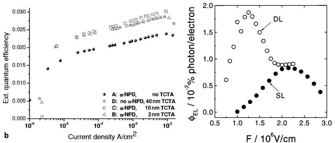
Slika 3.5: Lijevo: učinkovitost uređaja s Alq 3 |TCTA aktivnom granicom (A) i Alq 3 | \alpha -NPD granicom (B,C,D). [21] Kod gustoća struje oko 10 -2 A/cm 2 , koje odgovaraju primjenjenom naponu većem od 5 V, učinkovitost se počinje smanjivati. Desno: učinkovitost jednoslojnog filma (smjesa TPD:PBD:PC) i dvoslojne diode (TPD:PC)|PBD, u ovisnosti o prosječnom polju u uređaju. [104]
