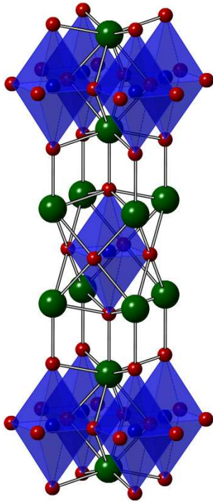
Slika 5.4: Kristalna struktura spoja \text{La}_{2-x}\text{Sr}_x\text{CuO}_4 .
