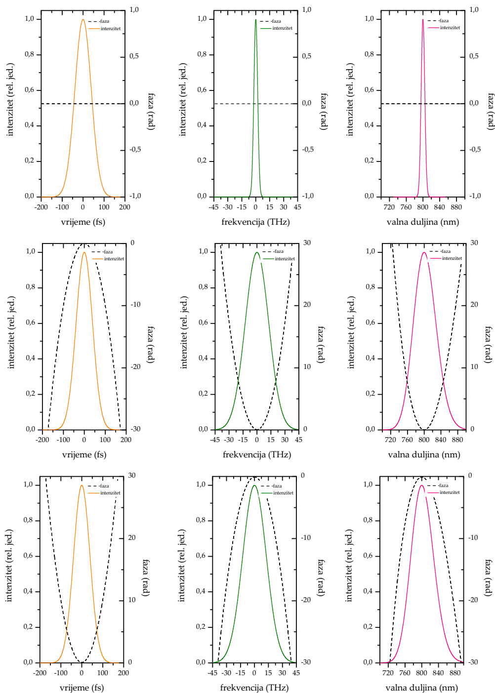
Slika 2.2: Utjecaj faze drugoga reda na intenzitet i fazu pulsa u vremenskoj i spektralnoj domeni te spektra pulsa u ovisnosti o valnoj duljini. Gore: Polje bez faze drugoga reda. Sredina: uključen pozitivni linearni cvrkuć iznosa -0.001 \text{ rad}/f s^2 . Dolje: uključen negativni linearni cvrkuć iznosa 0.001 \text{ rad}/f s^2 . Puls je centriran na 800 \text{ nm} sa anvelopom Gaussovog oblika te vremenskim trajanjem od \tau_p=92 \text{ fs} što odgovara spektralnoj širini od \approx 10 \text{ nm} (FWHM).
