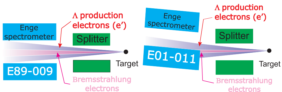
(a) Engage konfiguracija u eksperimentu E89-009 (b) Engage konfiguracija u eksperimentu E01-001.
