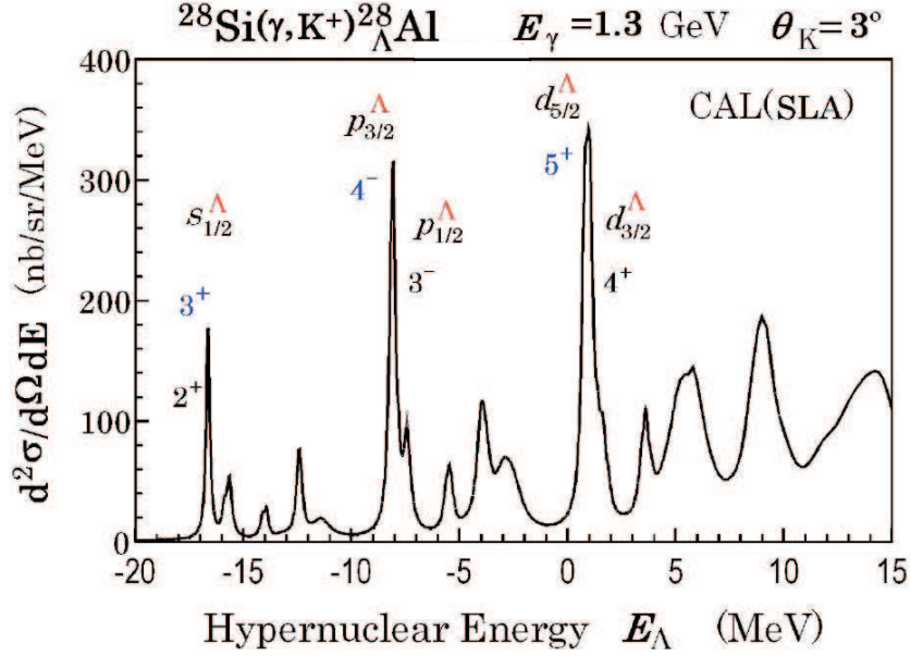
SLIKA 5.7: TEORIJSKI PREDVIĐEN SPEKTAR ZA ^{28}\text{Si}(\gamma, K^+)\Lambda^{28}\text{Al} REAKCIJU. RAČUN JE RAĐEN S E_\gamma = 1.3 \text{ GeV} I \theta_{K^+}^{LAB} = 3^\circ U SLA IZOBARNOM MODELU [31] [33].
