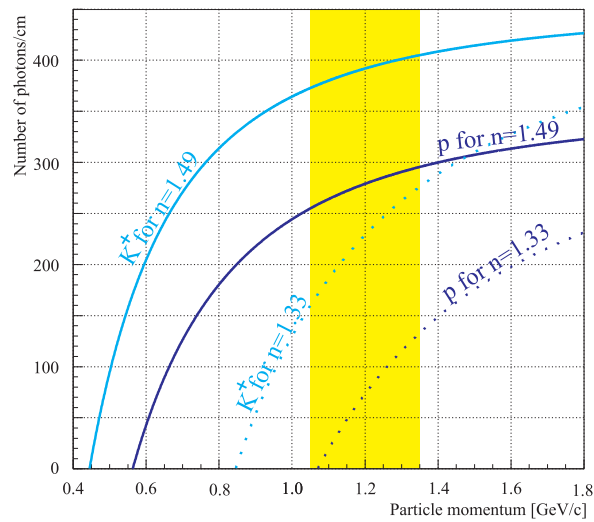
SLIKA 2.13: OVISNOST BROJA PRODUCIRANIH FOTOELEKTRONA U ČERENKOVljevim detektorima o impulsu kaona i protona za dva različita radiatora: voda ( n=1.33 ) i akrilni radiator ( n=1.49 ). Obojano područje reprezentira impulsnu akceptanciju HKS-A.
