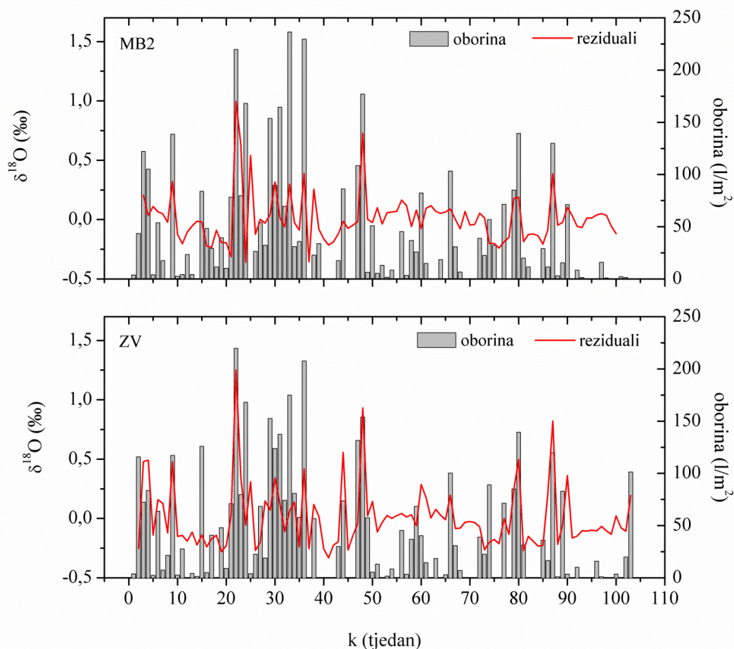
Slika 4.3.30. Reziduali vremenskih nizova vrijednosti \delta^{18}\text{O} za Zvir i bunar 2 u Martinšćici s tjednom količinom oborine na postaji Klana (DHMZ).
