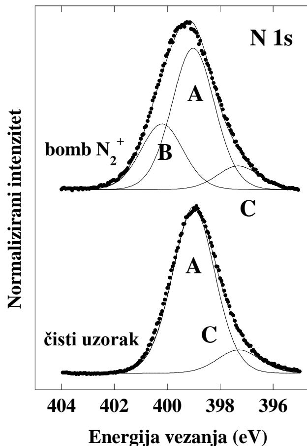
Slika 5.20: Fotoemisijски spekter oko N 1s orbitale mjereno na čistoj BN nanocjevčici i uzorku bombardiranom 4 min ionima N_2^+ energije 2 keV. Numerička prilagodba eksperimentalnih krivulja pomoću Voigtovih funkcija je prikazana punom linijom.
