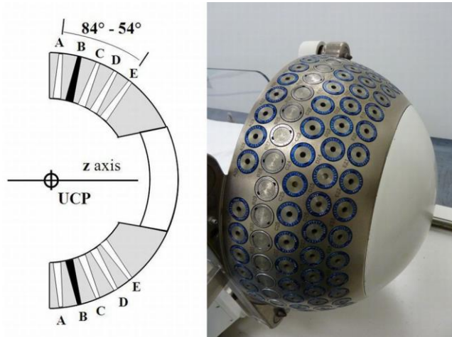
Slika 2.28 Kolimatorska kaciga gama noža s blokiranim kolimatorima prstena B (44 kolimatora potpuno blokirana). Ovakva konfiguracija fotonskih snopova odgovara mjerenom signalu detektora M_2 .
