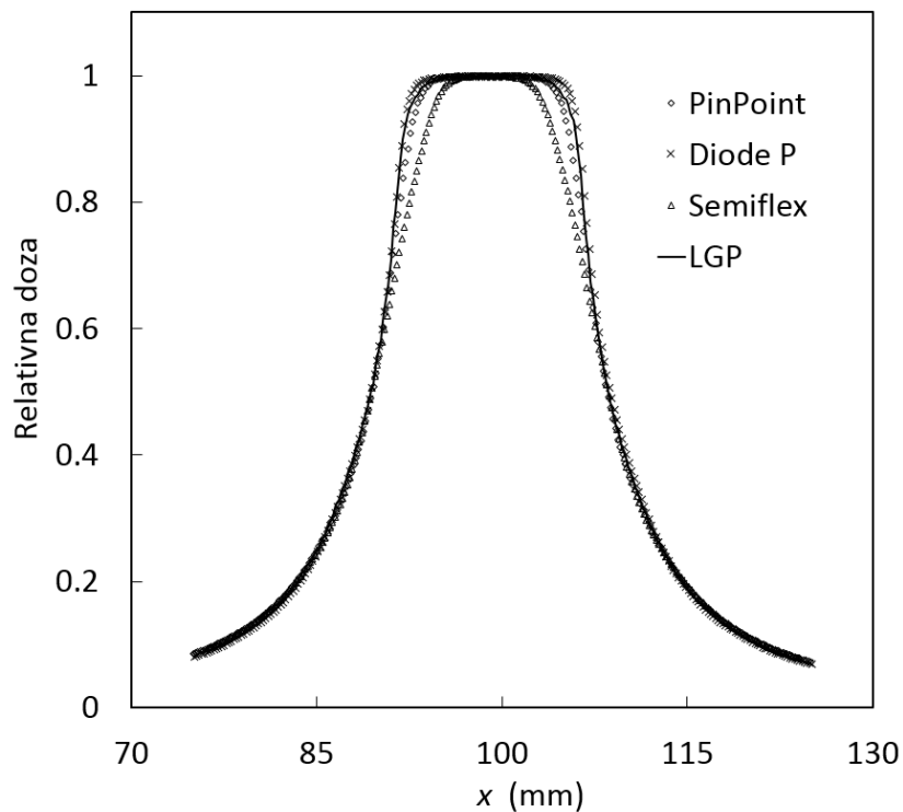
Slika 3.3 Usporedba LL-profila doze za 18 i 14 mm-ski kolimator mjenjenih ionizacijskim komorama PinPoint i Semiflex te poluvodičkim detektorom Diode P s računalno simuliranim LL-profilima (LGP).
