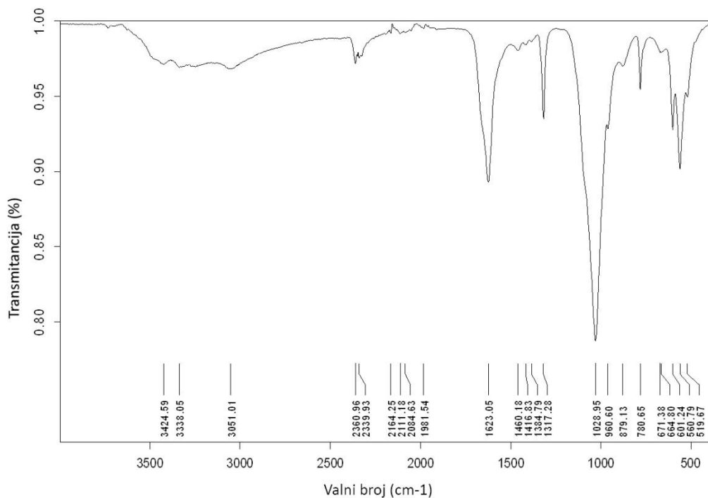
Slika 20. FT-IR spektar uzorka OS4b. (ATR), \tilde{\nu}_{\max} / \text{cm}^{-1} : 3333 (O-H istezanje), 1623 (C=O istezanje), 1317 (C-O istezanje), 1028 ( \text{PO}_4^{3-} istezanje), 519 (O-C-O istezanje).
