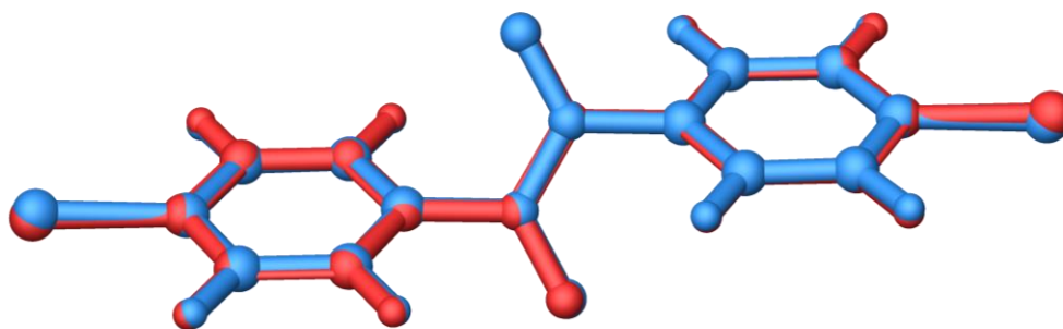
Slika 28. Preklapanje optimizirane geometrije (crvene boje) s geometrijom jedinične molekule u kristalu (plave boje) dimera p -bromnitrozobenzena. Atomi u azodioksidnoj vezi definirani su kao N4 i OM (RMSD vrijednost za sve atome iznosi 0,0587).
