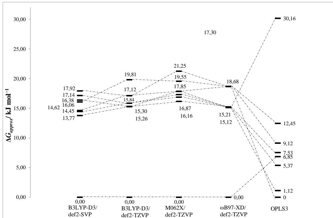
Slika D8. Relativne Gibbsove energije konformera azodioksida 2-nitrozopiridina uz kvazianharmoničku aproksimaciju izračunate na različitim razinama teorije.
