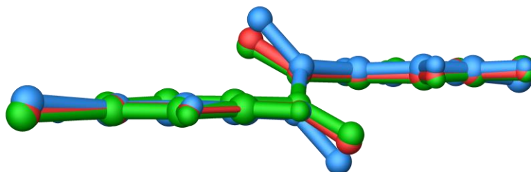
Slika 29. Preklapanje geometrija optimiziranih B3LYP-D3/def2SVP (zelene boje) i B3LYP-D3/def2TZVP (crvene boje) metodom s geometrijom jedinične molekule u kristalu (plave boje) dimera p -bromnitrozobenzena.
