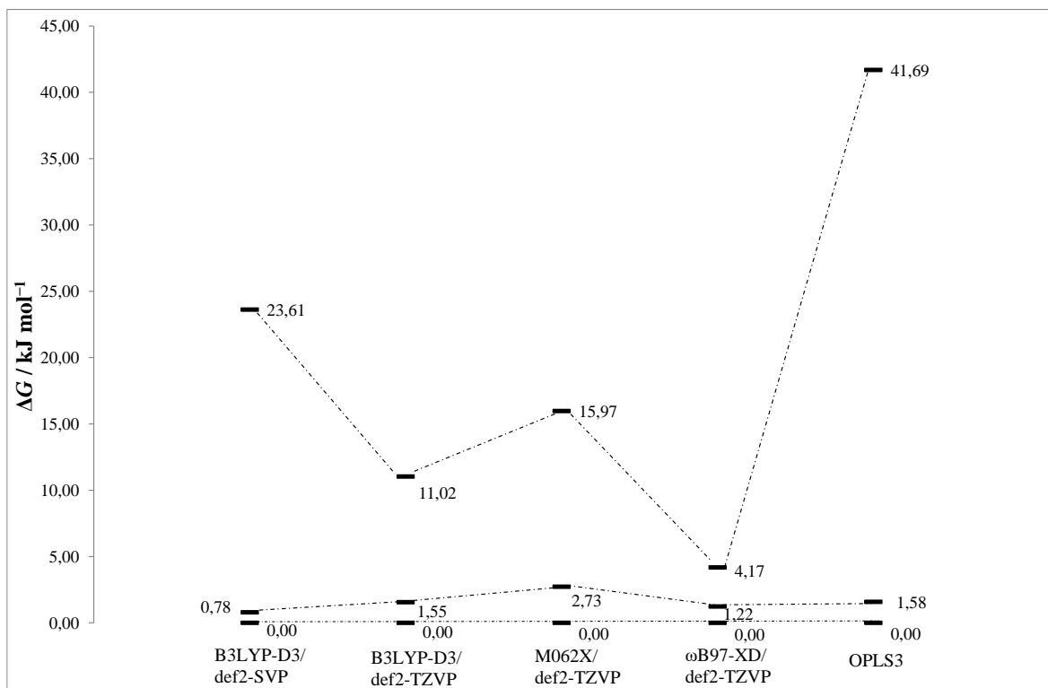
Slika D3. Relativne Gibbsove energije konformera azodioksida nitrobenzena izračunate na različitim razinama teorije.
