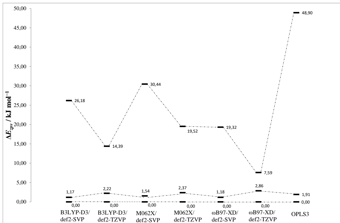
Slika 31. Relativne energije konformera azodioksida p -bromnitrozobenzena korigirane za energiju nulte točke izračunate na različitim razinama teorije.
