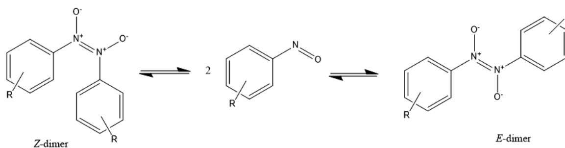
Slika 3. Monomer-dimer ravnoteža aromatskih C-nitrozo spojeva.
