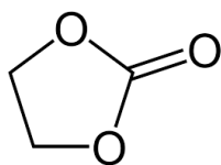
a) Etilen karbonat (EC)
