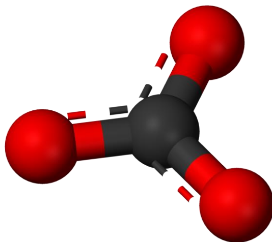
Slika 1. Prikaz strukture karbonatnog iona
