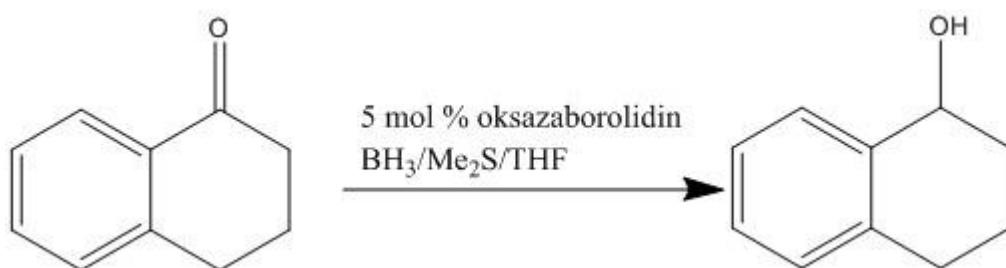
Shema 11. Općenita reakcija redukcije tetralona s boranom u otapalima THF i Me 2 S s oksazaborolidinom kao katalizatorom reakcije
