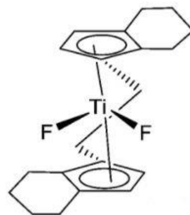
Slika 12. Etilen bis( \eta^5 -tetrahidroindenil)titanij difluorid
