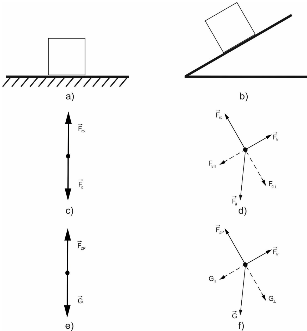
Slika 3.3. a) tijelo na ravnoj podlozi; b) tijelo na kosini; c) dijagram sila na tijelo koje se nalazi na ravnoj podlozi; d) dijagram sila na tijelo koje se nalazi na kosini; e) dijagram sila na ravnu podlogu; f) dijagram sila na podlogu kosine
