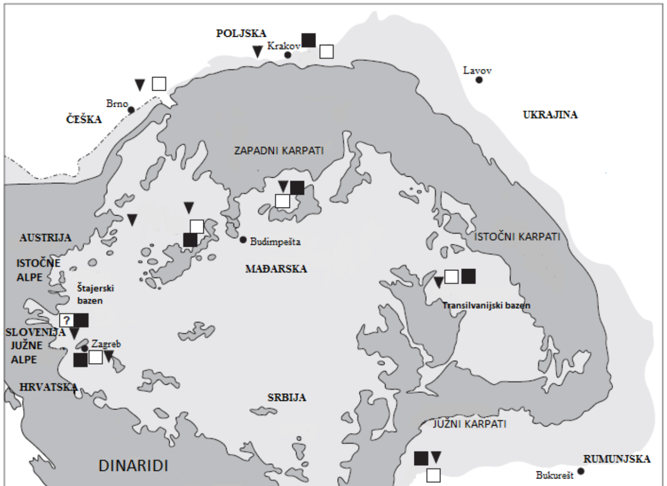
Slika 21. Distribucija pteropoda Clio fallauxi (bijeli kvadrati), Clio pedemontana (crni kvadrati) i Vaginella austriaca (crni trokut) unutar Centralnog Paratethysa (prema Bošnjak et al., 2017).
