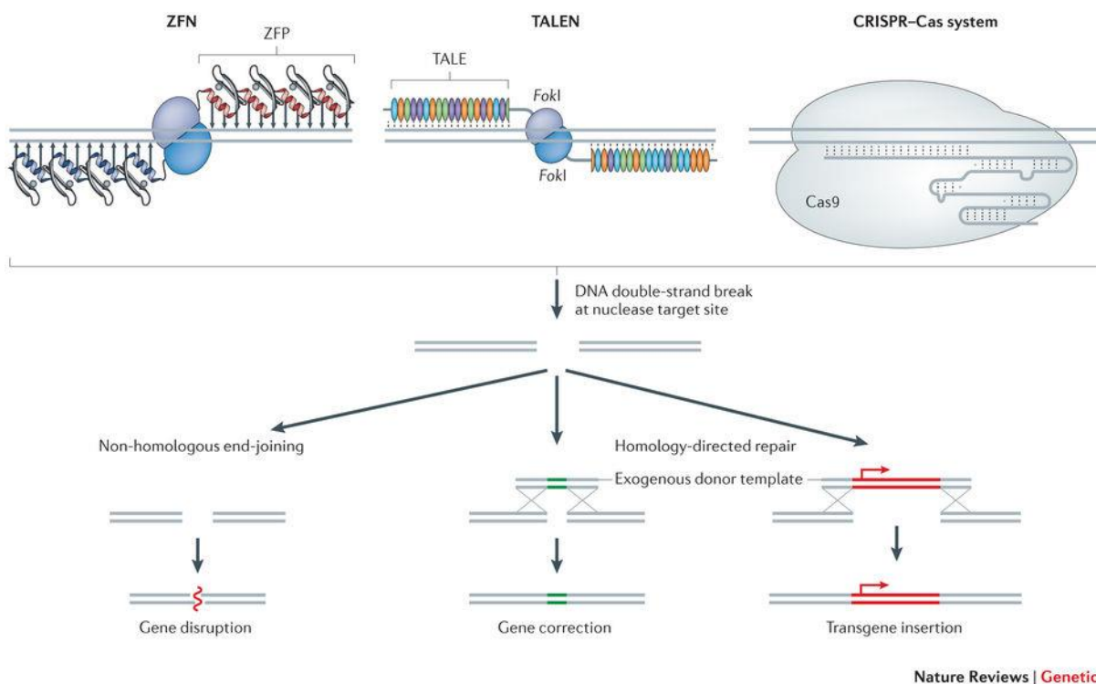
Slika 2. Usporedba ZFN, TALEN, i CRISPR/Cas sustava. (Yin i sur. 2014)
