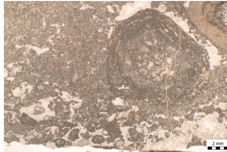
Slika 24: Cijanobakterijska gruda
