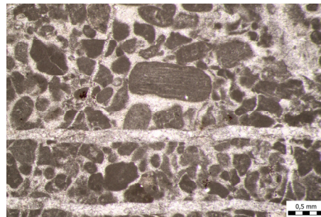
Slika 45: Favreina salevensis
