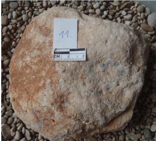
Slika 48: Rudistni vapnenac
