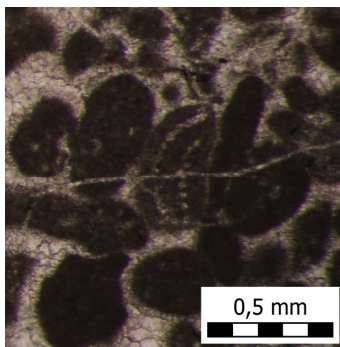
Slika 46: Favreina salevensis
