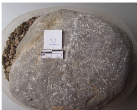
Slika 11: Valutica permskog vapnenca s mikrofosilima
