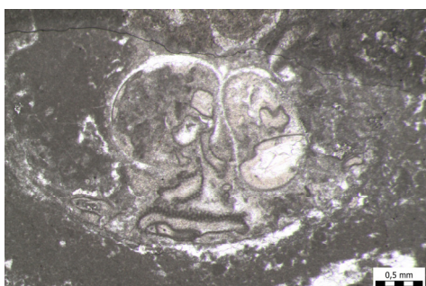
Slika 39: Presjek puža
