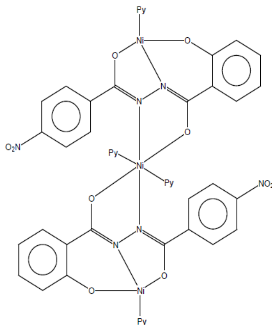
Slika 9. Hidrazon kao didentatni ligand
