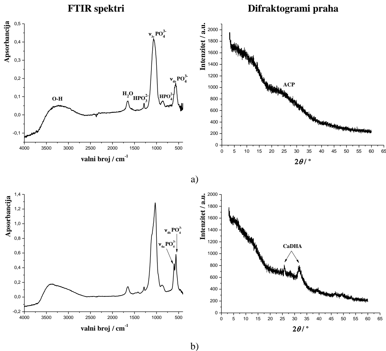
Slika 18. FTIR spektri i difraktogrami prača taloga nastalog u kontrolnom sustavu nakon: a) 10 min, b) 30 min i c) 60 min. Početne koncentracije reaktanata iznose c(\text{CaCl}_2 \cdot 2 \text{H}_2\text{O}) = c(\text{Na}_2\text{HPO}_4) = 5 \text{ mmol dm}^{-3} i c(\text{NaCl}) = 0,15 \text{ mol dm}^{-3} . Eksperimentalni uvjeti: magnetsko miješanje pri 25 °C i \text{pH}_{\text{poč}} 7,4 .
