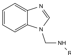
Slika 15. Strukturna formula N -supstituiranih derivata benzimidazola 16
