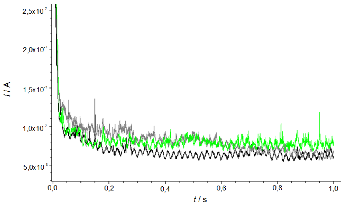
Slika 63. Tri uzastopna kronoamperograma u disperziji s nepoznatom veličinom i koncentracijom NČ Au u 0,1 \text{ mol dm}^{-3} \text{NaNO}_3 na potencijalu od 1,0 \text{ V} (vs. \text{Ag/AgCl} ), t = 1 \text{ s} uz t_s = 0,0002 \text{ s} .
