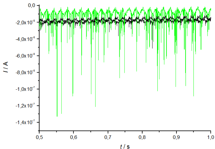
Slika 56. Kronoamperogram snimljen u originalnim uzorku s dubine od 10 m RJ 03/2016. (crna krivulja) i nakon provedene djelomične oksidacije uzorka (zelena krivulja) zakisljeni do pH = 2, E = -0,8 V t = 2 s uz t_s = 0,0004 s
