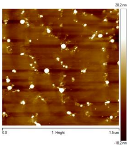
Slika 48. AFM topografski 3D (a, c) i 2D (b,d) prikaz visina uzoraka disperzije \text{Fe}^{2+} i \text{HS}^- 5 \times 10^{-5} \text{ mol dm}^{-3} u 0,55 \text{ mol dm}^{-3} , veličina oslikane površine: 2,5 \mu\text{m} \times 2,5 \mu\text{m} (a,b) i 1,5 \mu\text{m} \times 1,5 \mu\text{m} (c,d)
