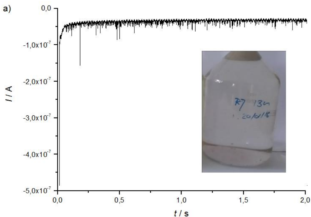
Slika 57. a) Kronoamperogram uzorka RJ s dubine od 13m 03/2016. zakisljeni do pH = 2, E = -0,8 V, t = 2 s uz t_s = 0,0004 s
