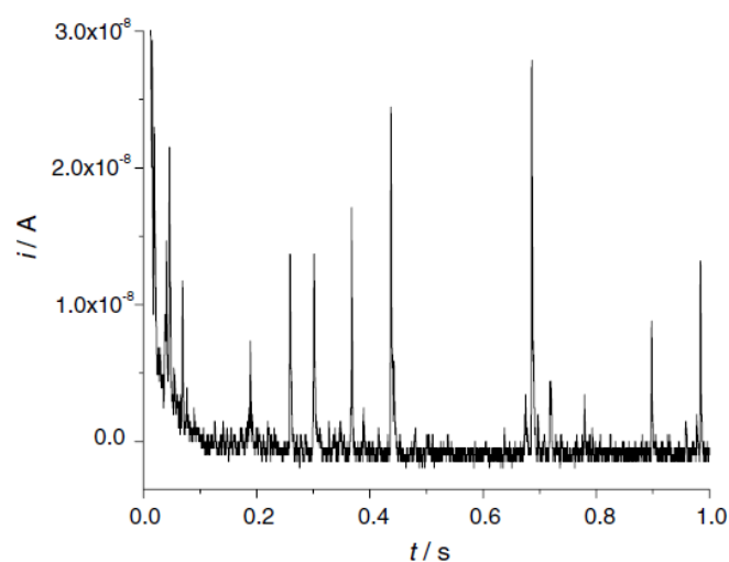
Slika 7. Kronoamperometrija suspenzije montmorilonita (0,2 g dm -3 ) u 0,1 M KCl-u (Scholz i sur., 2004)
