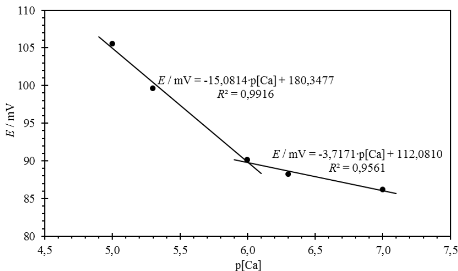
Slika 4.24. Baždarni dijagram kalcijeve ISE bez miješanja reakcijske smjese - ovisnost elektromotivnosti članka sačinjenog od kalcijeve ISE i kombinirane elektrode o negativnom logaritmu koncentracije \text{Ca}^{2+} iona u otopini pri 25\text{ }^{\circ}\text{C} , \text{pH} = 5,0 \pm 0,1 i I_c \approx 1 \times 10^{-3} \text{ mol dm}^{-3} koja je održavana stalnom pomoću NaCl. Baždarni dijagram je napravljen prema podacima iz tablice D2.
