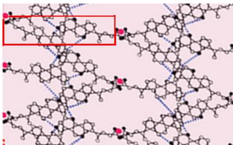
Slika 113. Prikaz dvoslojnog pakiranja (crveno) kolatnog kompleksa sintetiziranog iz NaCh i LaCl 3 . Ružičasto su obojani atomi lantana, crno atomi kisika, a bijelo atomi ugljika. 114
