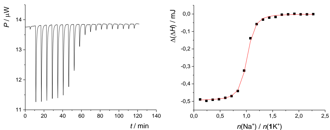
Slika 20. Mikrokalorimetrijska titracija \mathbf{K1}^+ ( c(\mathbf{1}) = 1,84 \times 10^{-4} \text{ mol dm}^{-3} , c(\mathbf{K}^+) = 5,12 \times 10^{-4} \text{ mol dm}^{-3} ) s \text{NaClO}_4 ( c = 2,10 \times 10^{-3} \text{ mol dm}^{-3} ) u metanolu pri \vartheta = 25,0 \text{ }^\circ\text{C} . a) Termogram; b) Ovisnost sukcesivnih promjena entalpije o omjeru množine reaktanata. ■ eksperimentalne vrijednosti, — izračunane vrijednosti.
