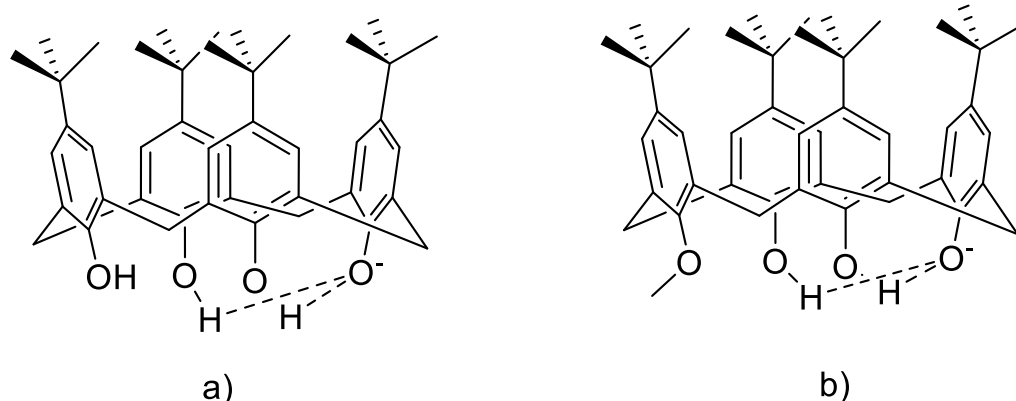
Slika 6. Vodikove veze u monoanionu a) nefunkcionaliziranog i b) monoalkiliranog kaliks[4]arena. 15
